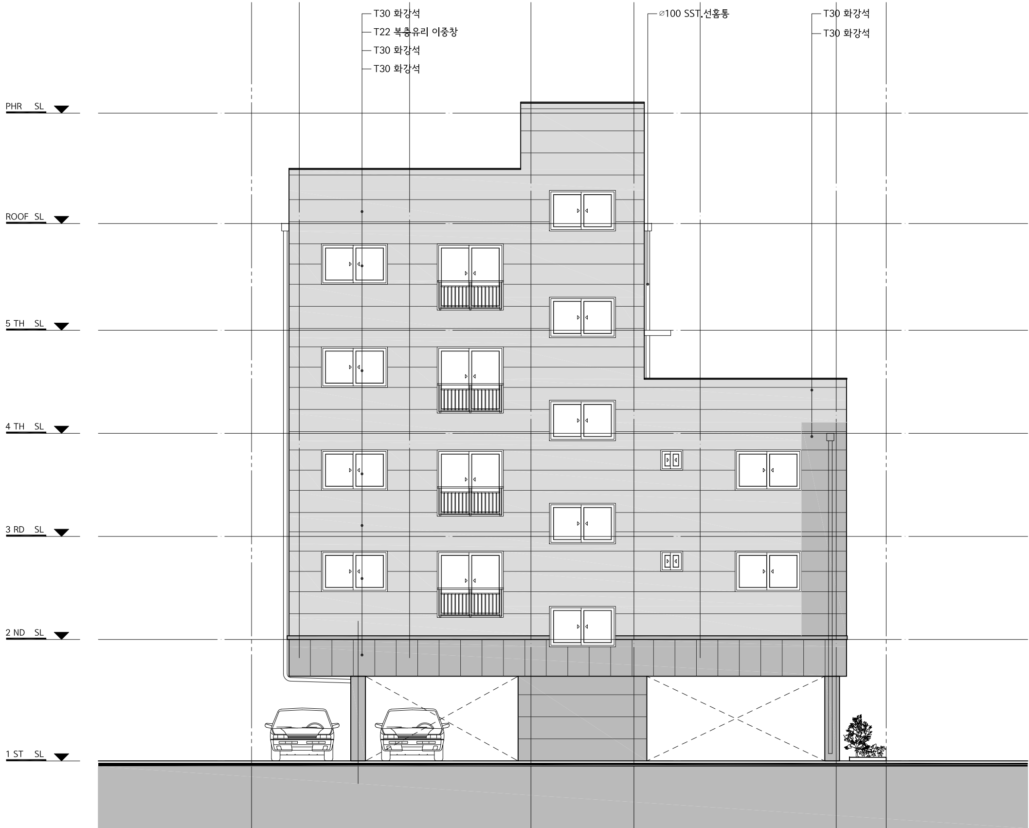
배면도 (남측) 축척 : 1/ 100
