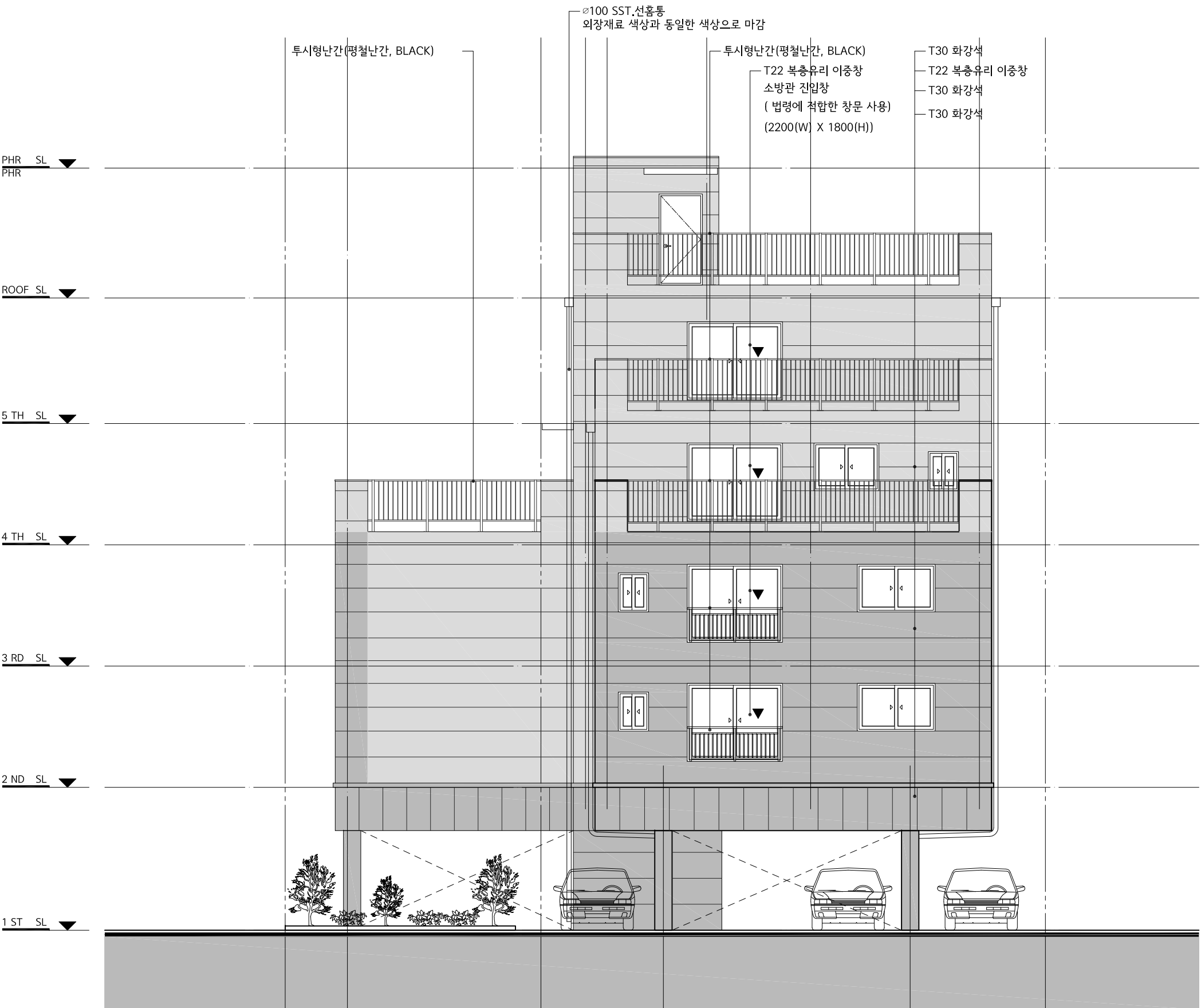
정면도 (북측) 축척 : 1/ 100
