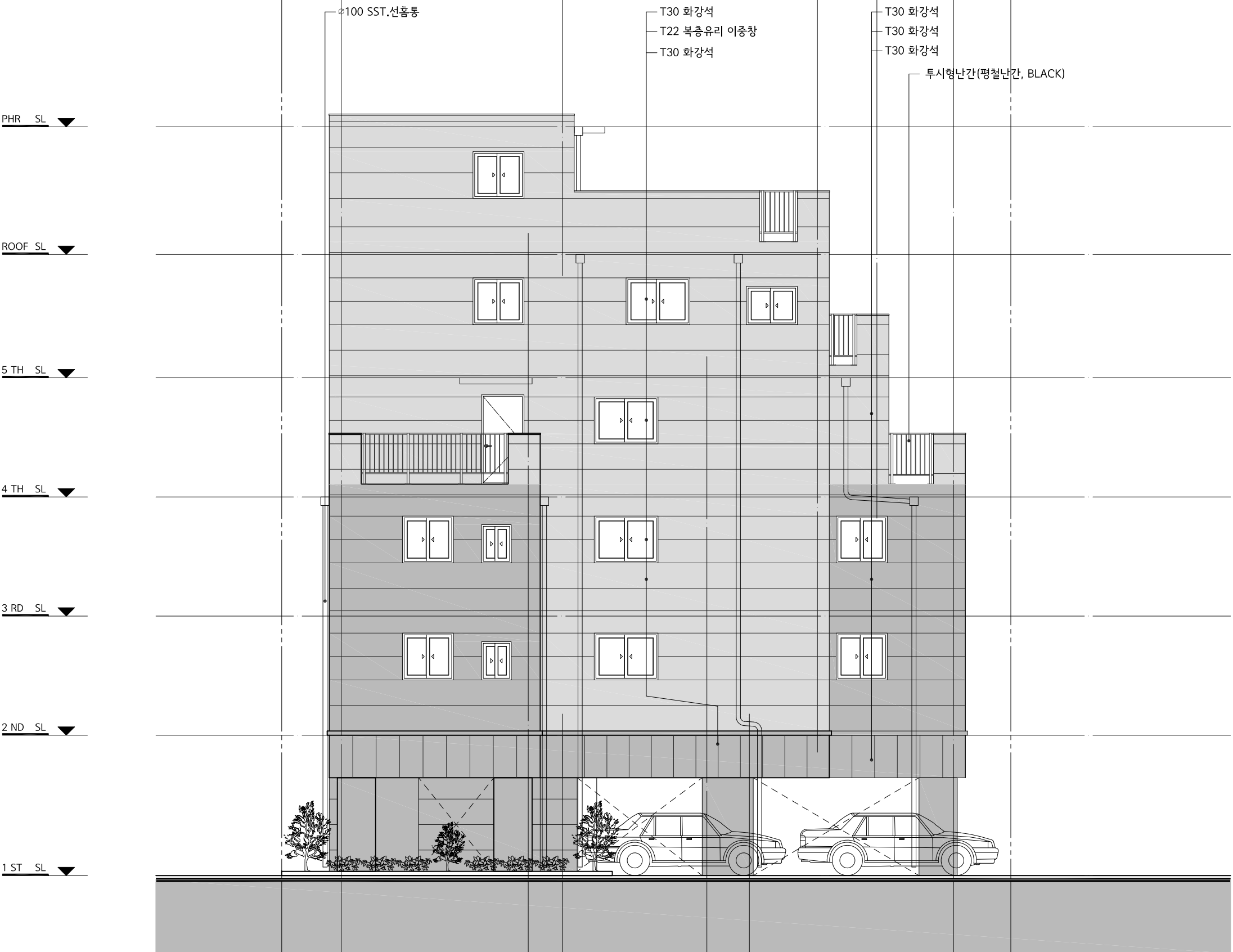
1 A 00 좌측면도 (동측) 축척 : 1/ 100
