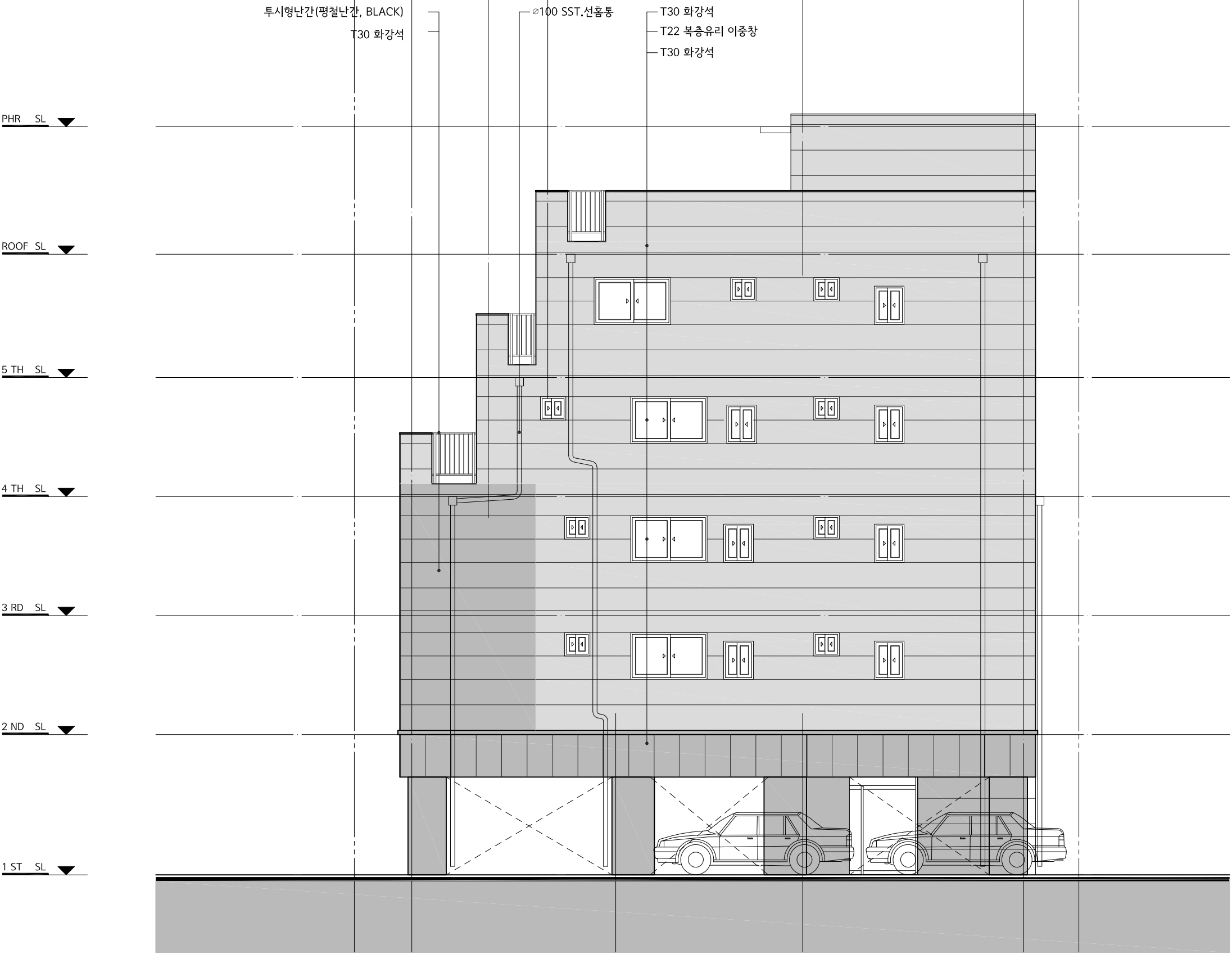
우측면도 (서측) 축척 : 1/ 100
